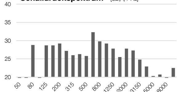
Schalldruckspektrum 5) [dB(A) / Hz]
